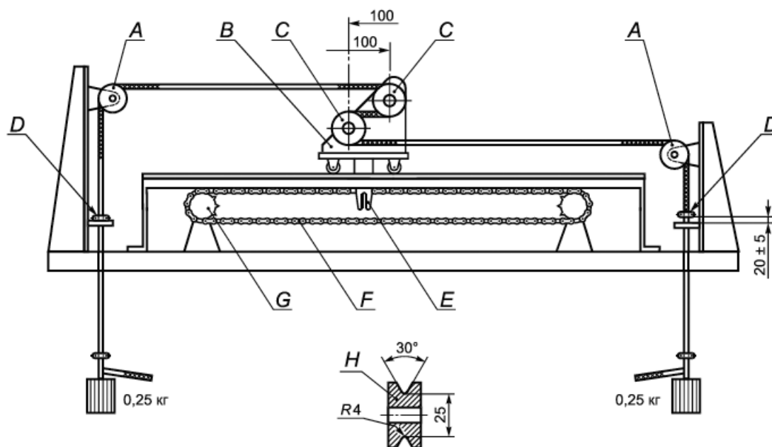
Рисунок 101 - Оборудование для испытания на изгиб для грелок для ног
